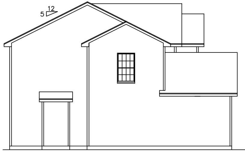
LEFT SIDE ELEVATION SCALE: 1/8" = 1'-0"
