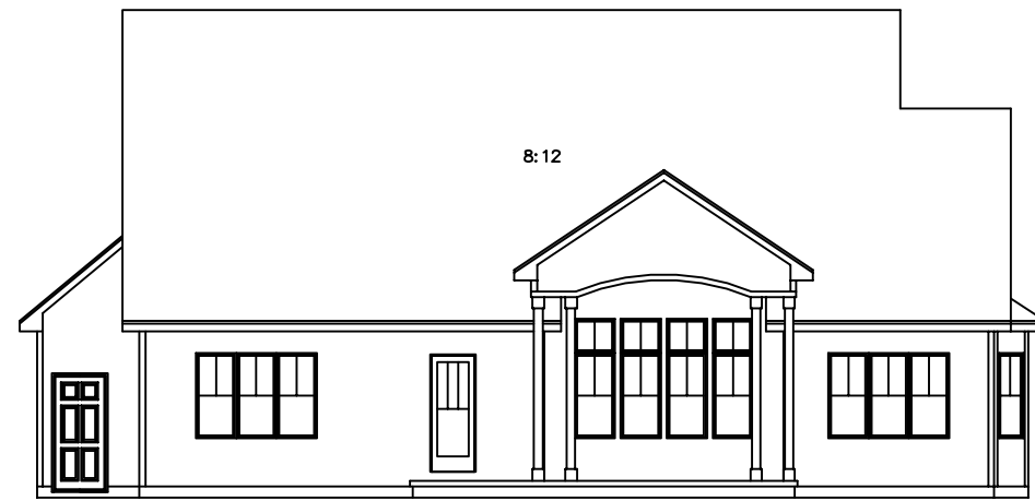
REAR ELEVATION SCALE: 1/8" = 1'-0"
